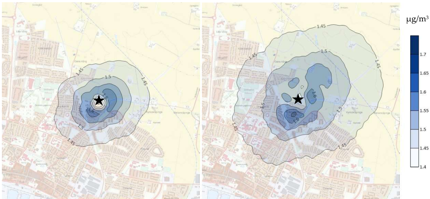
Figur 7. Totala halter av \text{SO}_2 beräknat som 98-percentil för timmedelvärden. Bilden till vänster visar scenario noll och bilden till höger visar scenario ett. Den svarta stjärnan visar placering av Östervångsverket.
