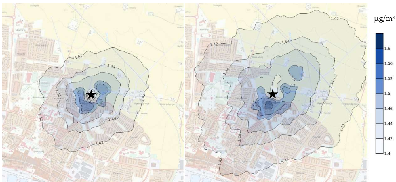
Figur 6. Totala halter av SO 2 beräknat som 98-percentil för dygnsmedelvärden. Bilden till vänster visar scenario noll och bilden till höger visar scenario ett. Den svarta stjärnan visar placering av Östervångsverket.
