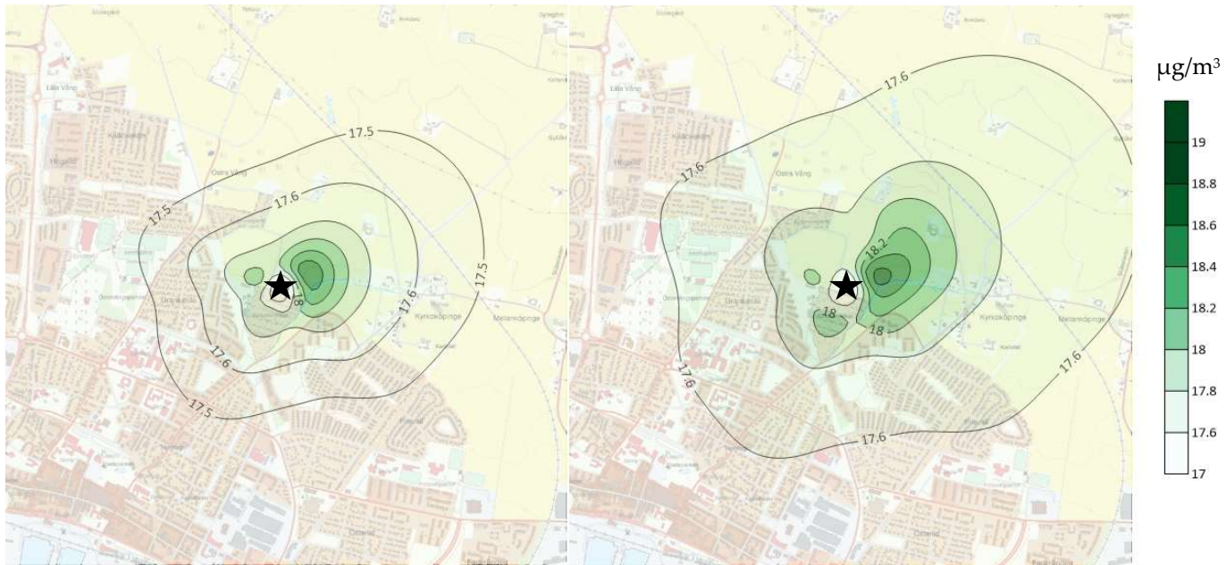
Figur 3. Totala halter av NO x beräknat som årsmedelvärde. Bilden till vänster visar scenario noll och bilden till höger visar scenario ett. Den svarta stjärnan visar placering av Östervångsverket.
