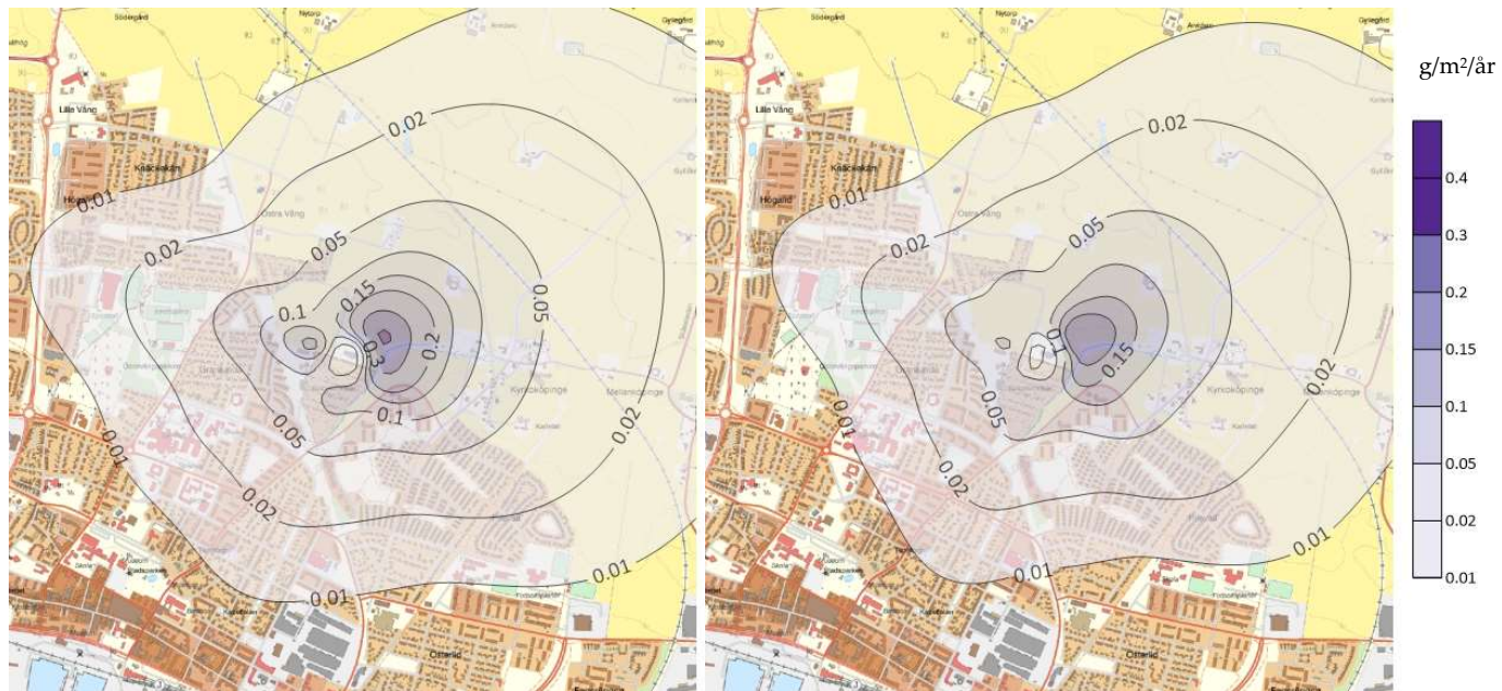
Figur 15. Beräknad totaldeposition av stoff [ \text{g}/\text{m}^2/\text{år} ]. Till vänster ses scenario noll och till höger scenario ett.
