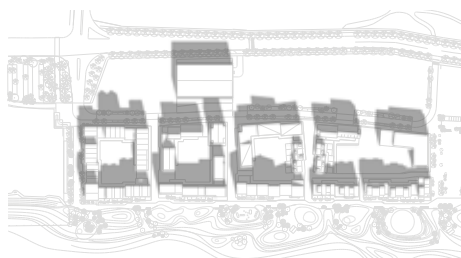
B. 12:00 Vårdagjämning 2022.03.20
