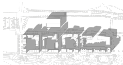
I. 15:00 Höstdagjämning 2022.09.23
