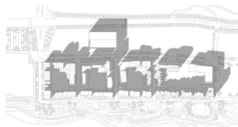
C. 15:00 Vårdagjämning 2022.03.20
