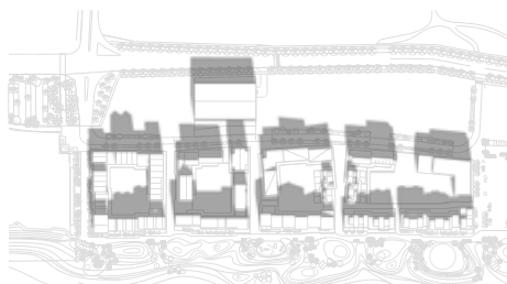
H. 12:00 Höstdagjämning 2022.09.23
