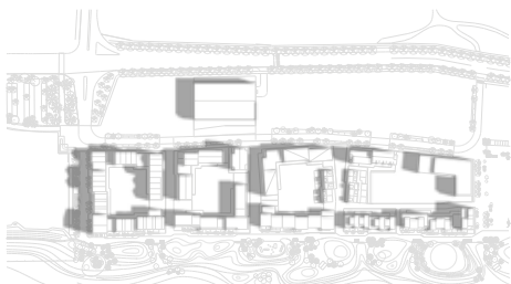
D. 09:00 Midsommardagen 2022.06.25
