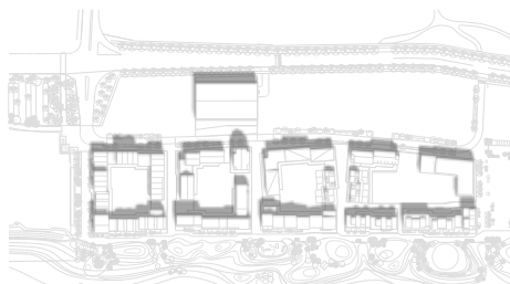
E. 12:00 Midsommardagen 2022.06.25
