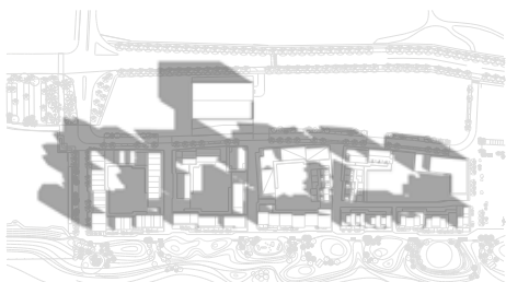
G. 09:00 Höstdagjämning 2022.09.23
