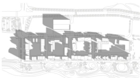
A. 09:00 Vårdagjämning 2022.03.20
