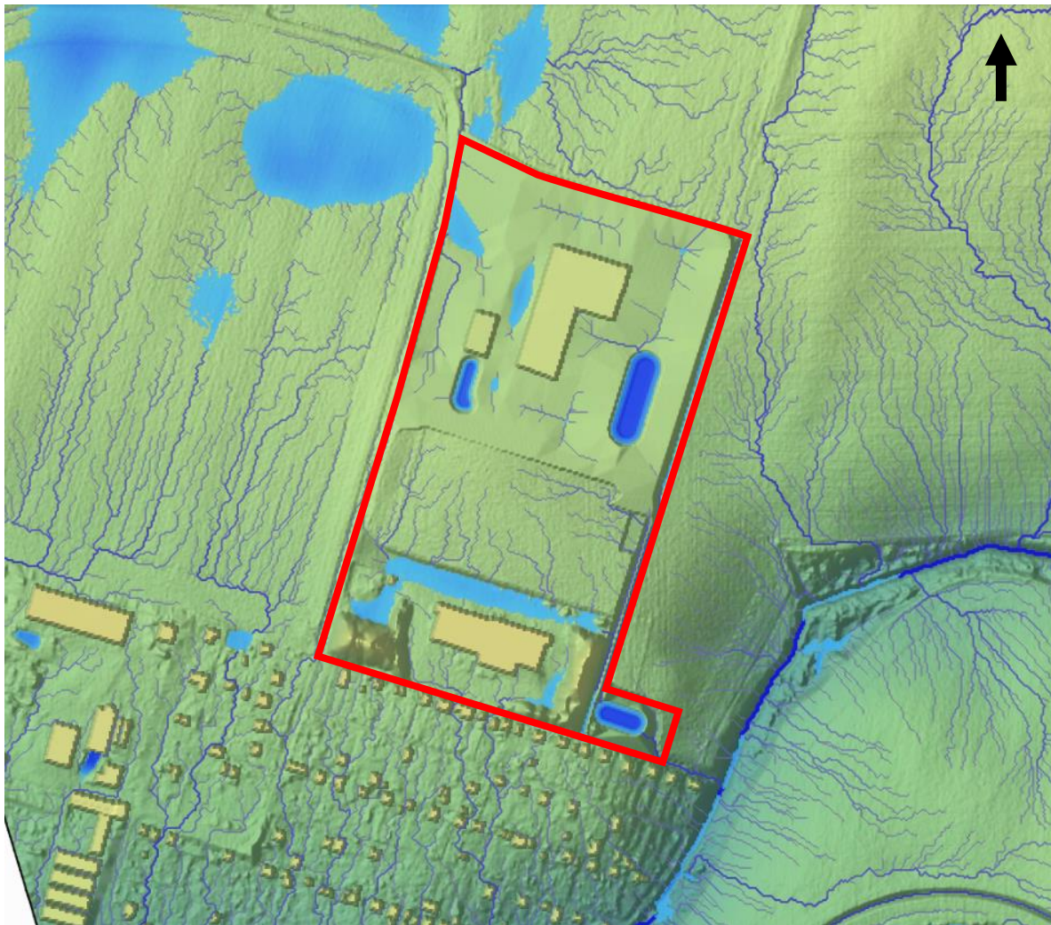
Figur 15. Förslag skyfallshantering i form av ny höjdsättning, dagvattendammar (fördröjning) och diken längs fastighetsgräns för ytlig avledning av flöden vid extrema regn. Bild erhållen från SCALGO Live 2023-03-23 efter modellering av ny höjdsättning och manuella tillägg av dagvattenledningar.
