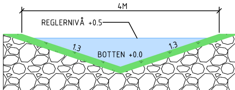
Figur 10. Principsektion för öppet med vegetationsbeklätt svackdike. Höjdangivelser avser relativa höjder från dikesbotten (nollplan).
